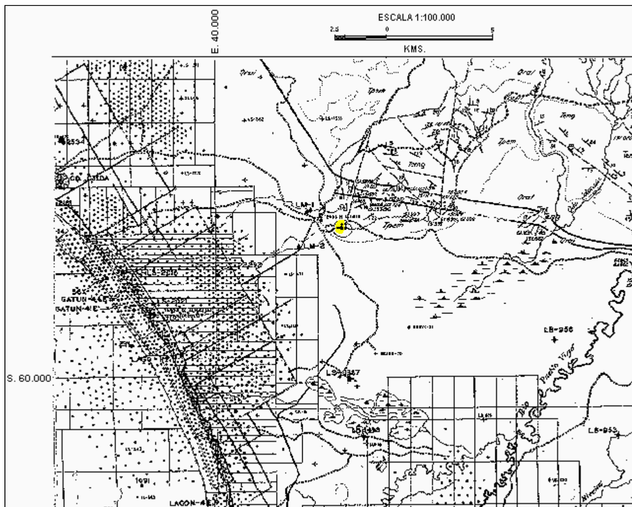
Tomado de: Geología de Superficie de la Creole Petroleum Corporation, Hoja D-3, 1967.
